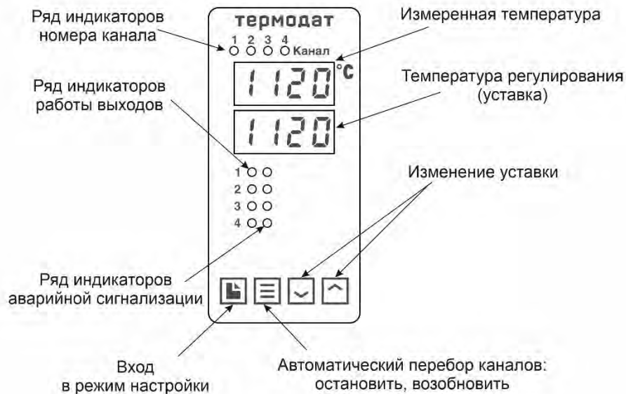
Рисунок 7 – Описание индикаторов и кнопок управления приборов 11М6-В...
