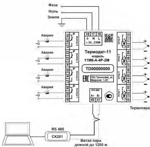
Рисунок 13 - Схема подключения Термодат -11М6-А... при использовании прибора как аварийного сигнализатора, напряжение питания 230В
