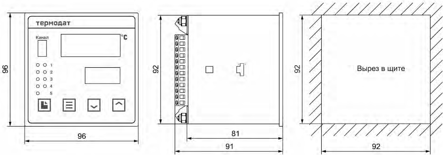
Рисунок 17 – Габаритные размеры прибора 11M6-A...
