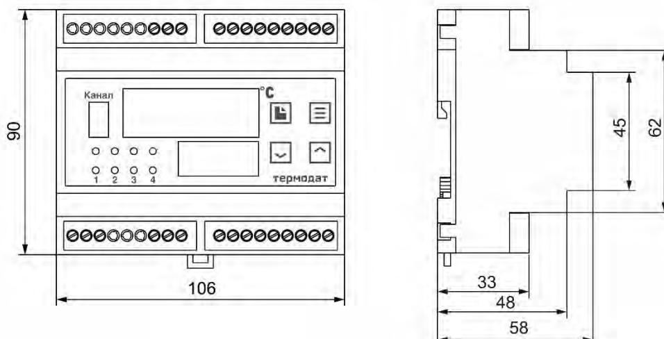
Рисунок 19 – Габаритные размеры прибора 11M6-P6...
