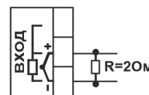
Токовый вход 0...40 мА
