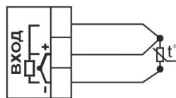
Термометр сопротивления
