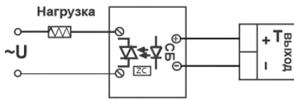
Управление однофазной нагрузкой с помощью блока СБ
