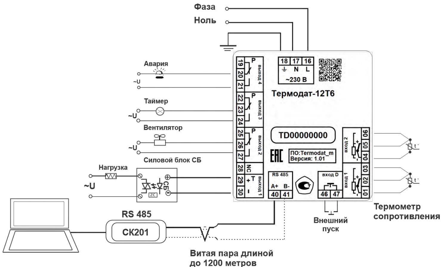
Рисунок 8 – Схема подключения прибора.
