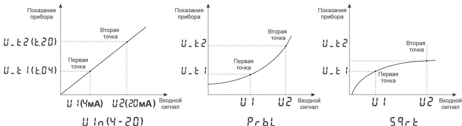
Рисунок 4 - Графики зависимости показаний прибора от входного сигнала при использовании входа типа U.in, PrbL, Sqrt и датчика 4...20
