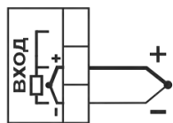
Термопара
