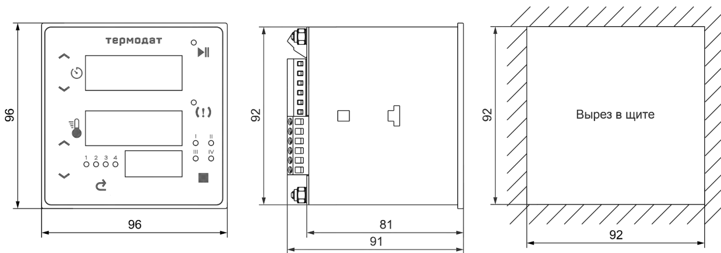
Рисунок 9 – Габаритные размеры прибора Термодат-12Т6
