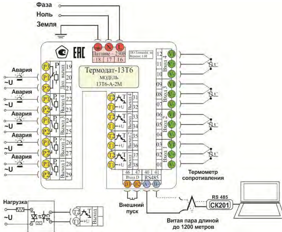
Рисунок 8.Схема подключения прибора.
