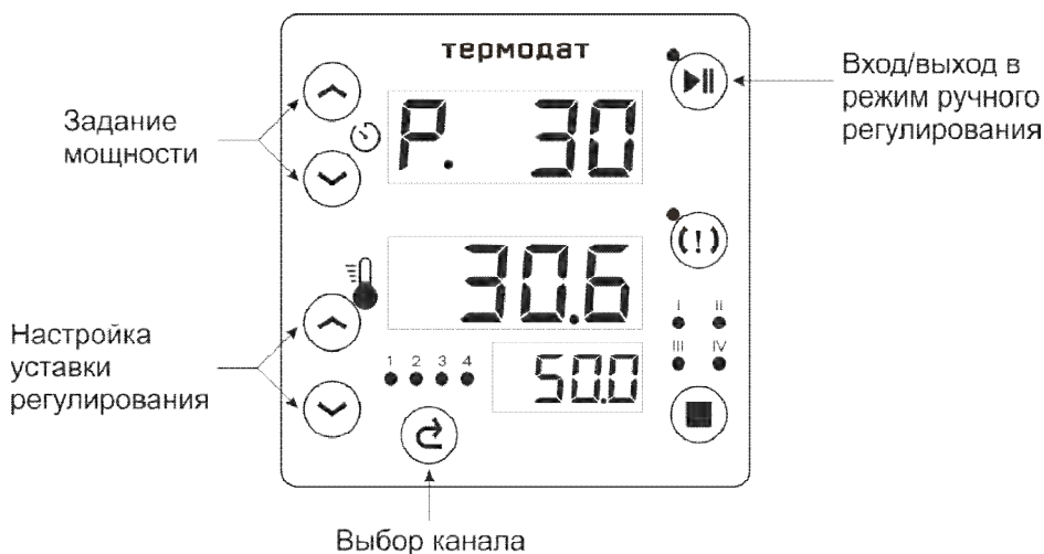
Рисунок 3. Ручное управление мощностью.
