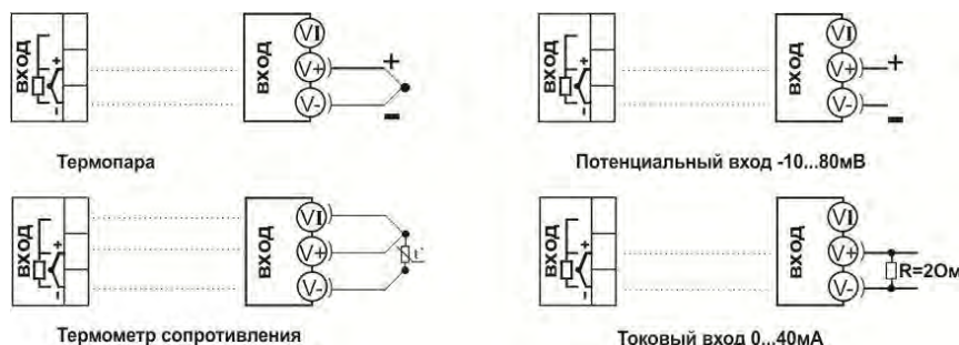
Рисунок 5.Схемы подключения датчиков.
