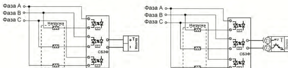
Подключение трехфазной нагрузки в шестипроводной схеме
