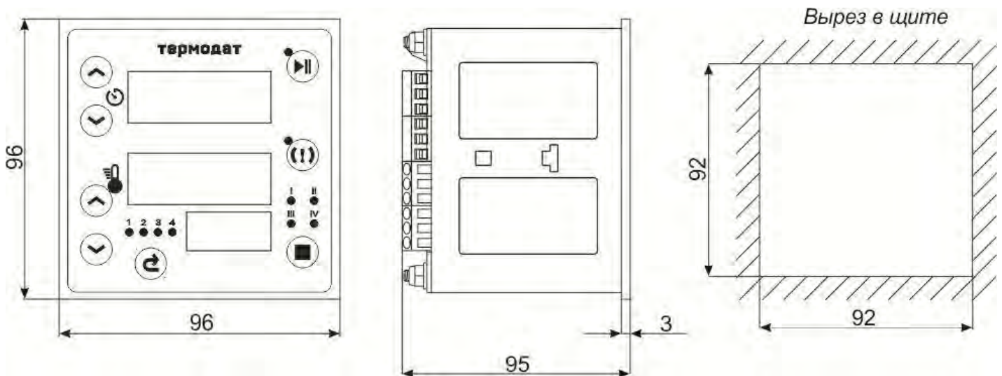
Рисунок 9.Габаритные размеры прибора Термодат-13Т6/...
