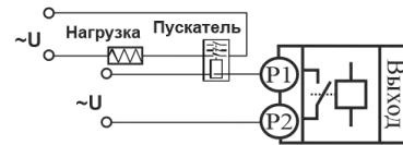
Подключение нагрузки мощностью более 2,3 кВт с помощью электромагнитного пускателя
