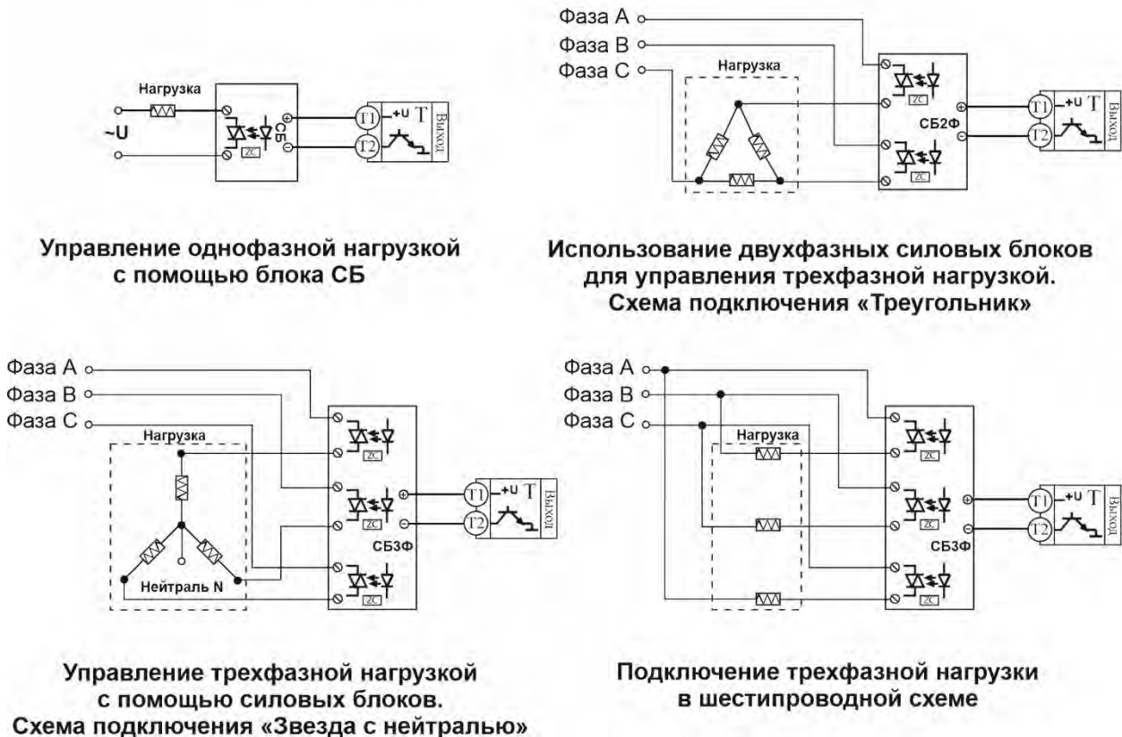
Рисунок 11 – Схемы подключения транзисторного выхода
