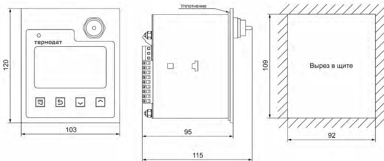
Рисунок 14 – Габаритные размеры основного блока прибора Термодат-25E6/..../F/IP67
