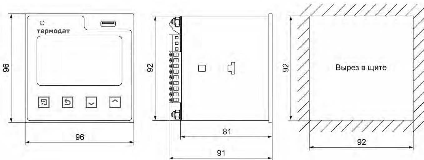
Рисунок 13 – Габаритные размеры основного блока прибора Термодат-25E6/..../F
