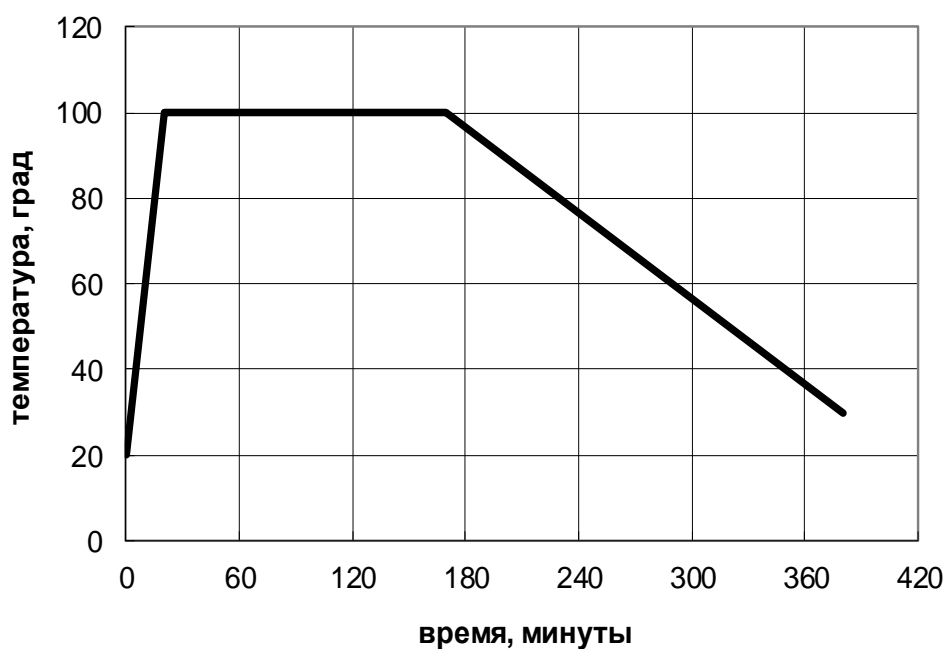
Рисунок 5–График режима термообработки
