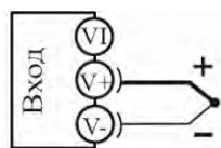
Термопара
