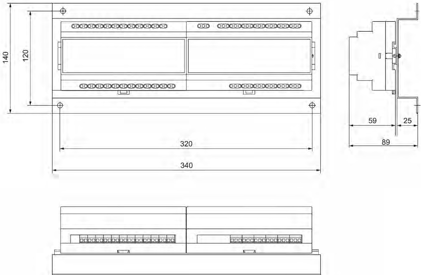
Рисунок 10 – Габаритные размеры блока измерения PB4/8UB(12UB)
