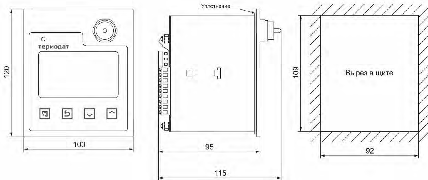
Рисунок 8 – Габаритные размеры прибора Термодат-25М6/...../F
