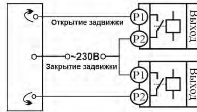
Подключение электрораздвижки
