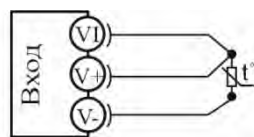
Термометр сопротивления
