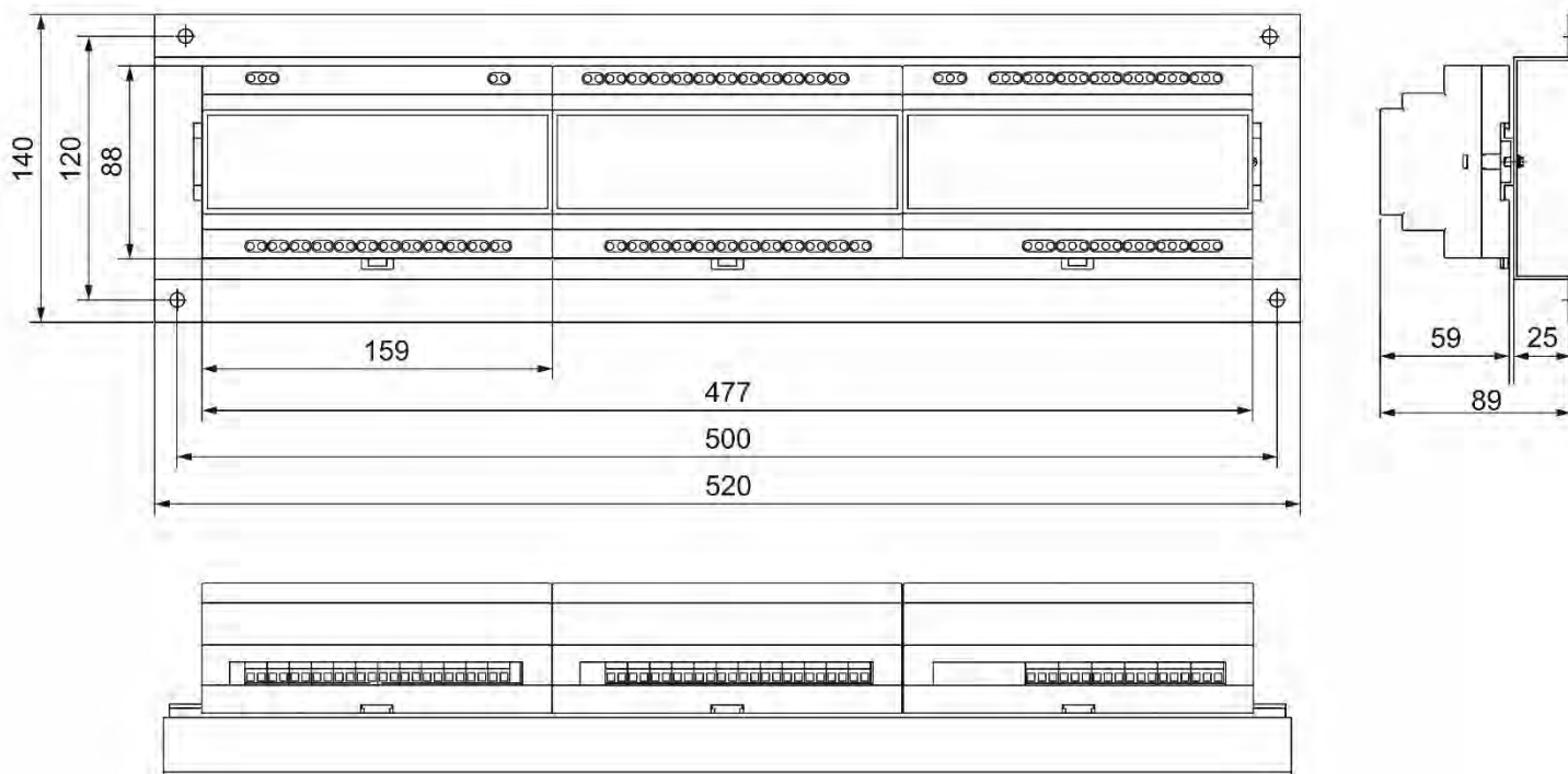
Рисунок 12 – Габаритные размеры блока измерения, блока выходов и блока аналоговых выходов РВ/12УВ/12Р/12Р-12А
