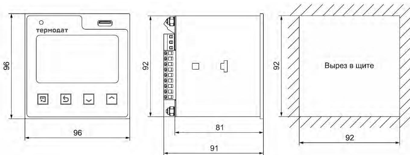
Рисунок 8 – Габаритные размеры прибора Термодат-25М6/...../F
