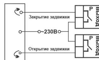
Подключение электроздвижки
