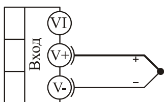
термопара
