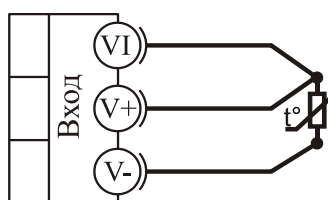
термометр сопротивления
