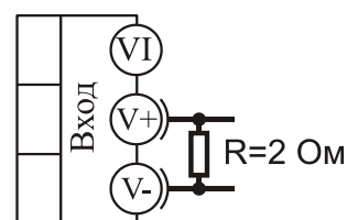
0...40 мА токовый вход
