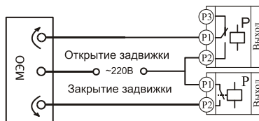
Подключение электрозадвижки
