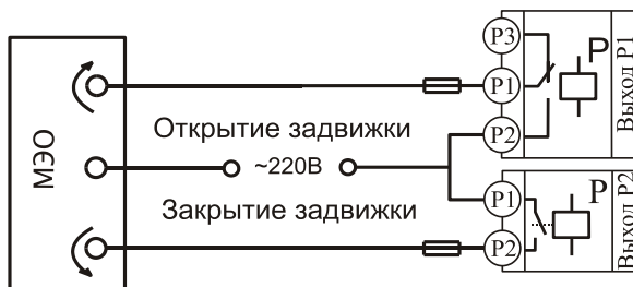
Подключение электрозадвижки
