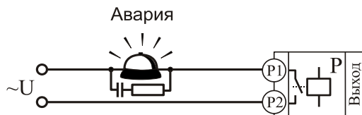
Подключение аварийной сигнализации
