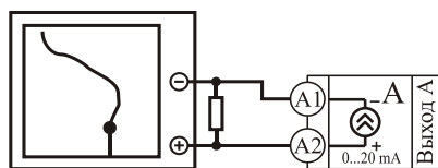
Подключение самописца
