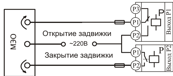
Подключение электрозадвижки
