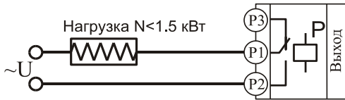
Подключение нагрузки менее 1,5 кВт
