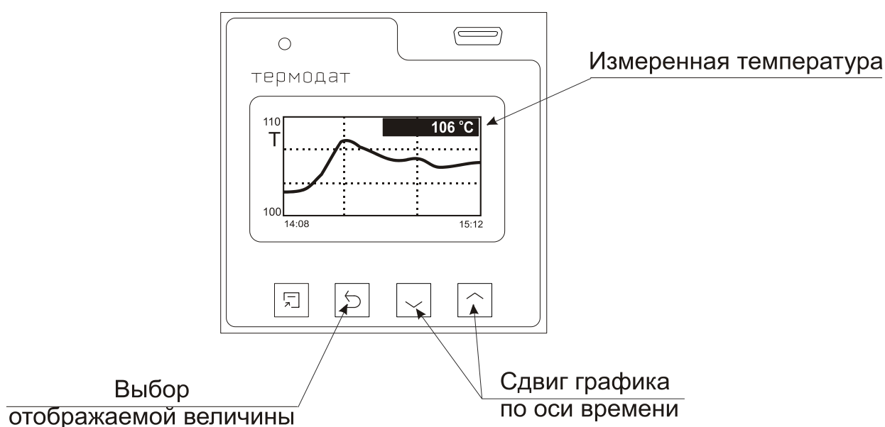
Рис. 2. Режим индикации «График»
