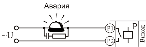
Подключение аварийной сигнализации
