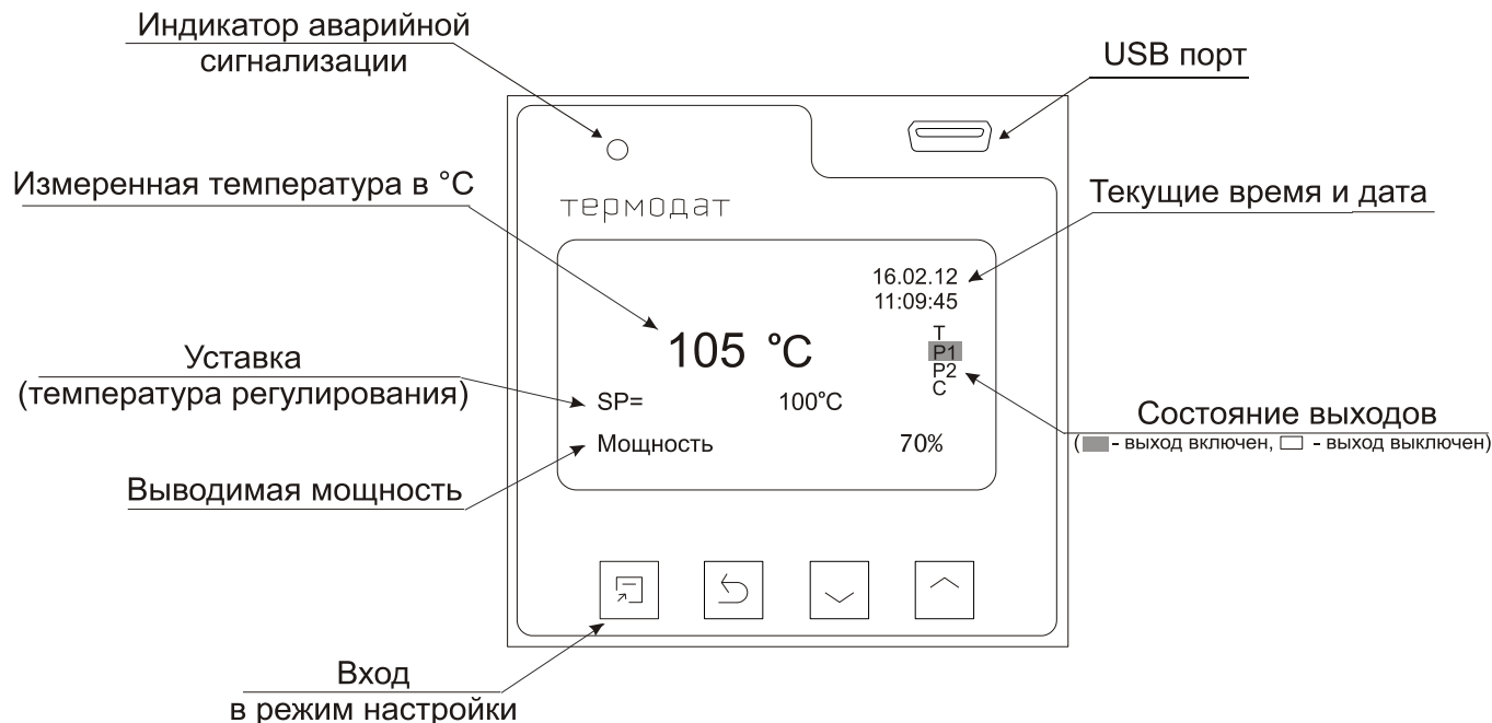
Рис. 1. Режим индикации «Текст»
