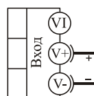
0...80 \text{ мВ} потенциальный вход
