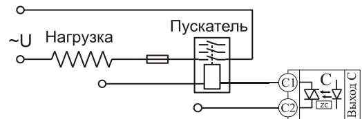
Подключение электромагнитного пускателя
