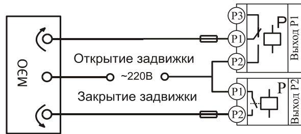
Подключение электрозадвижки
