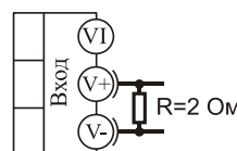
0...40 \text{ мА} токовый вход
