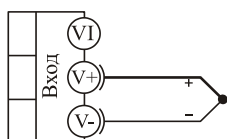
терморпара
