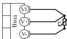
термометр сопротивления
