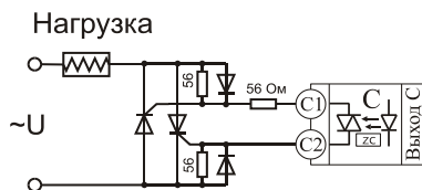
Подключение внешних тиристорov
