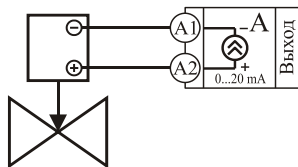
Подключение задвижки с электроприводом
