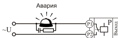
Подключение аварийной сигнализации
