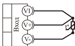
термометр сопротивления
