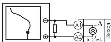
Подключение самописца
