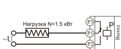
Подключение нагрузки менее 1,5 кВт
