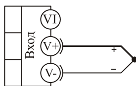
термопара
