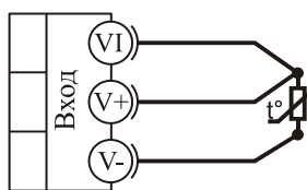
термометр сопротивления
