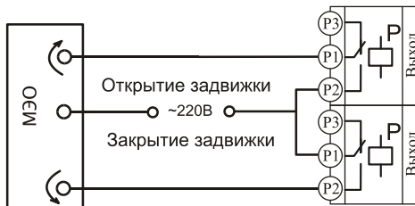
Подключение электрораздвижки
