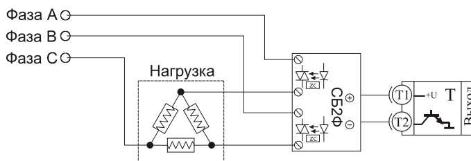
Использование двухфазных силовых блоков для управления трёхфазной нагрузкой. Схема подключения "Треугольник"
