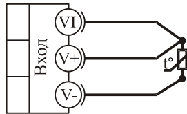
термометр сопротивления
