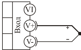
термопара
