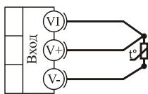
термометр сопротивления
