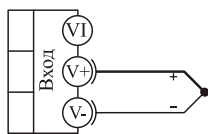
термопара
