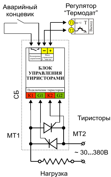
Схема подключения тиристоров к блоку управления
