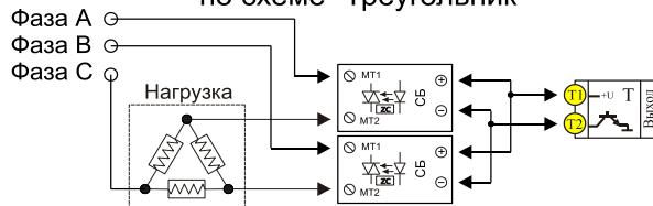
Подключение трехфазной нагрузки по схеме "Треугольник"
