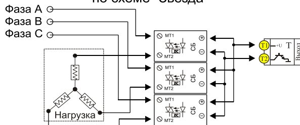
Подключение трехфазной нагрузки по схеме "Звезда"
